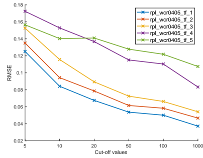
(b) RMSE WCrusbust0405.
